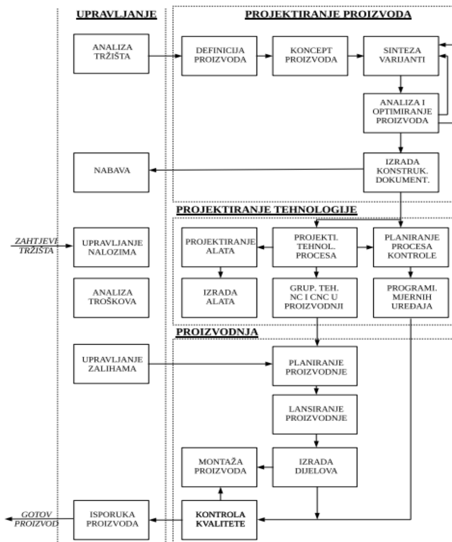
Slika 11. Elementi proizvodnog sustava [9]
