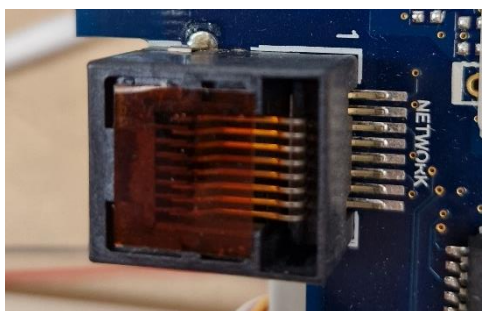
Slika 33. Spajanje rutera
