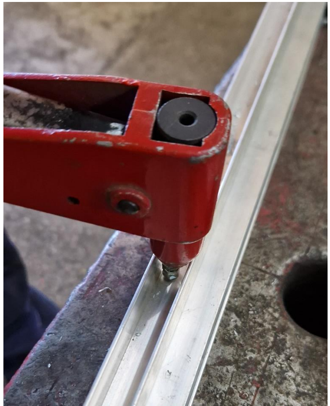
Slika 9. Zakivanje zakovica
