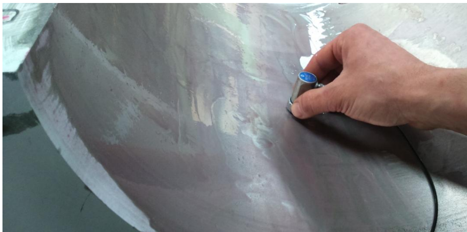
Slika 74: UZ ispitivanje donje polovice ležaja
