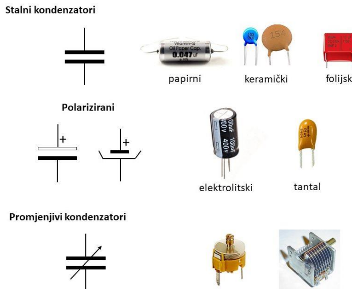
Slika 23. Vrste kondenzatora [28]
