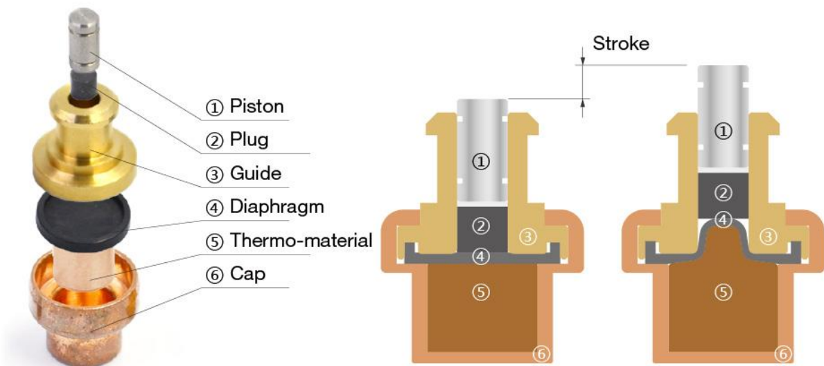
Slika 8. Termalni aktuator [16]
