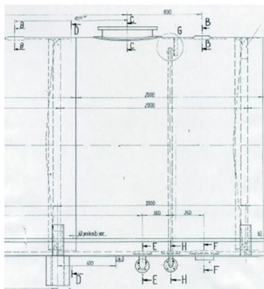
Slika 15. Shematski pregled priključaka tekuće i plinske faze [8]
