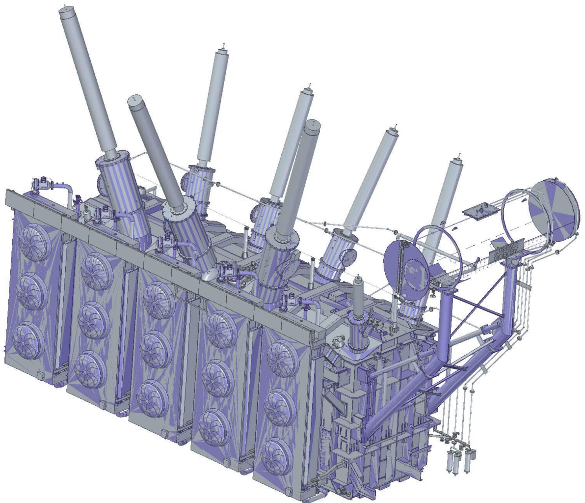
Slika 1. Primjer transformatora
