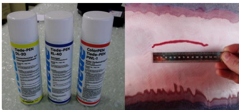
Slika 2.2. Ispitivanje penetrantima: razvijatelj, čistač i penetrant (lijevo) penetrantska indikacija (desno)
