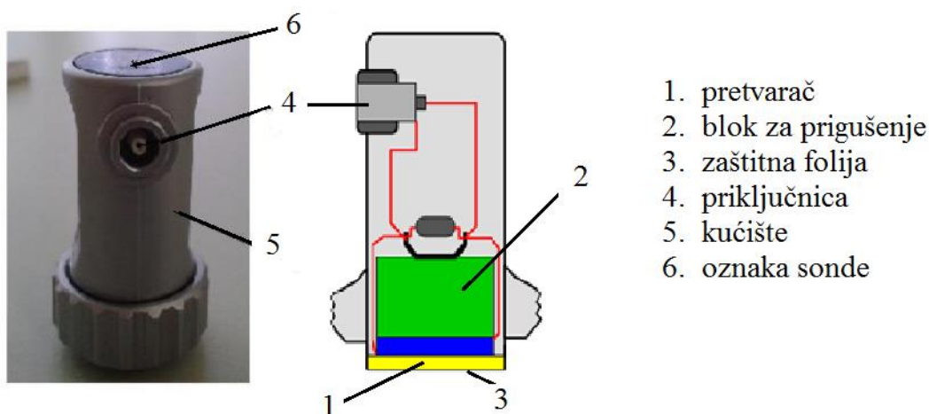
Slika 5.2. Ravna sonda
