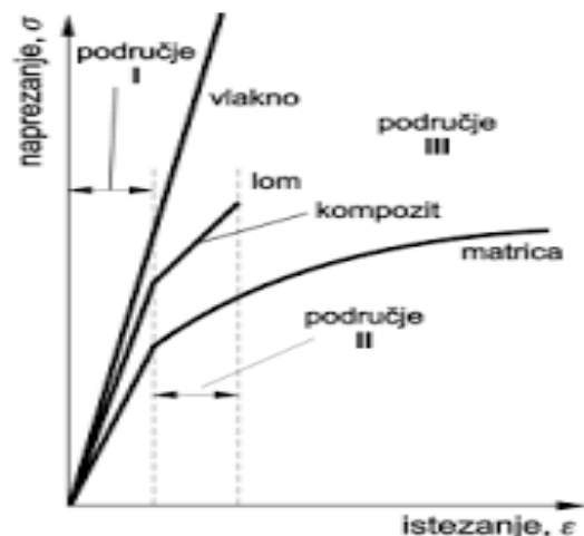
Slika 7. Dijagram naprezanje-istežanje vlaknima ojačan kompozit [13]
