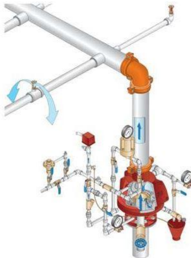
Slika 35. Predodžba shematski prikaz dijela mokrog sprinkler sustava
