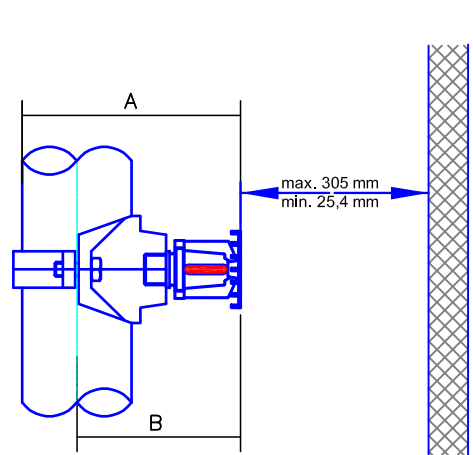
Detalj 3 SPRINKLERI MUZIČKA STUČICA
