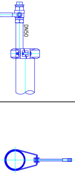
Detalj 1 Prilika za sprinkl
