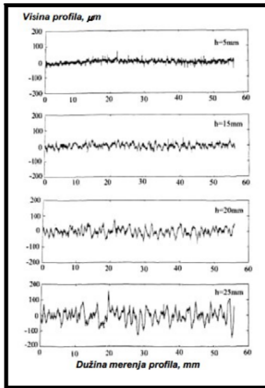
Slika 6.3. Primjeri obrađene površine u ovisnosti od dubine reza h [6]
