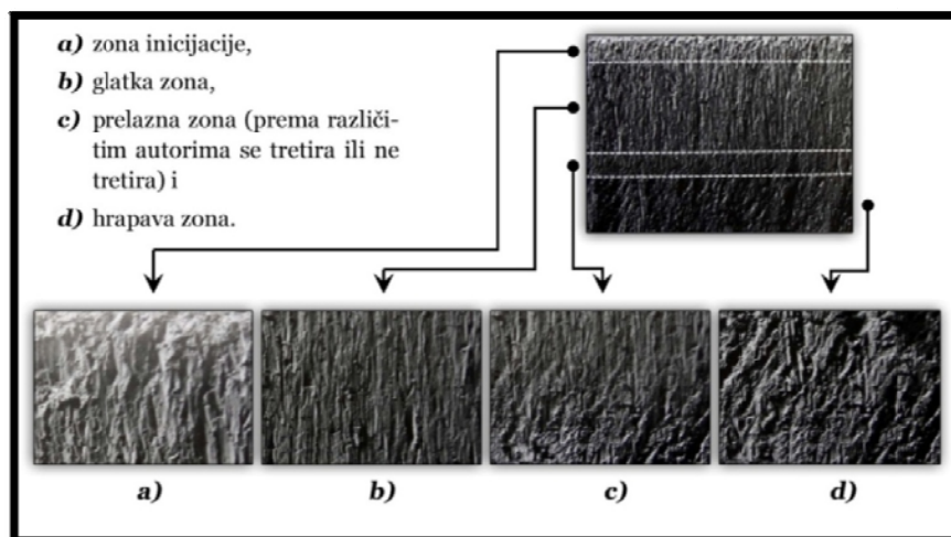
Slika 6.4. Mikro struktura rezne površine [12]
