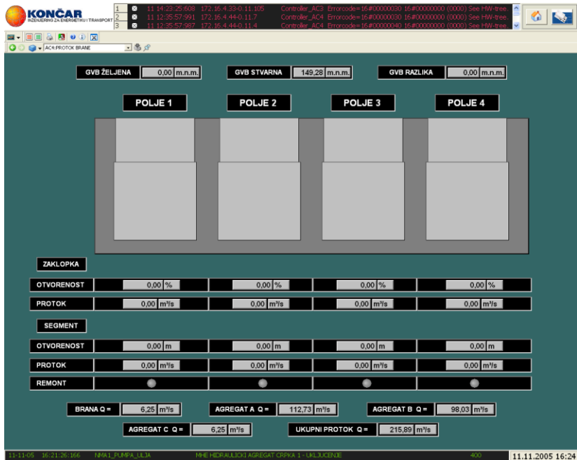
Slika 15. Protok brane
