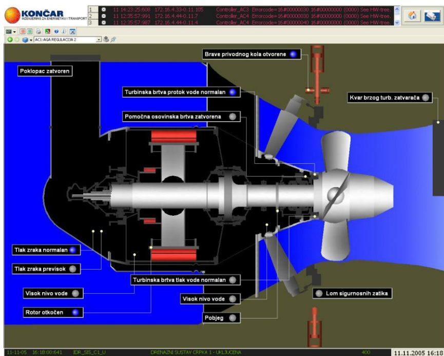
Slika 10. Signali regulacije 1
