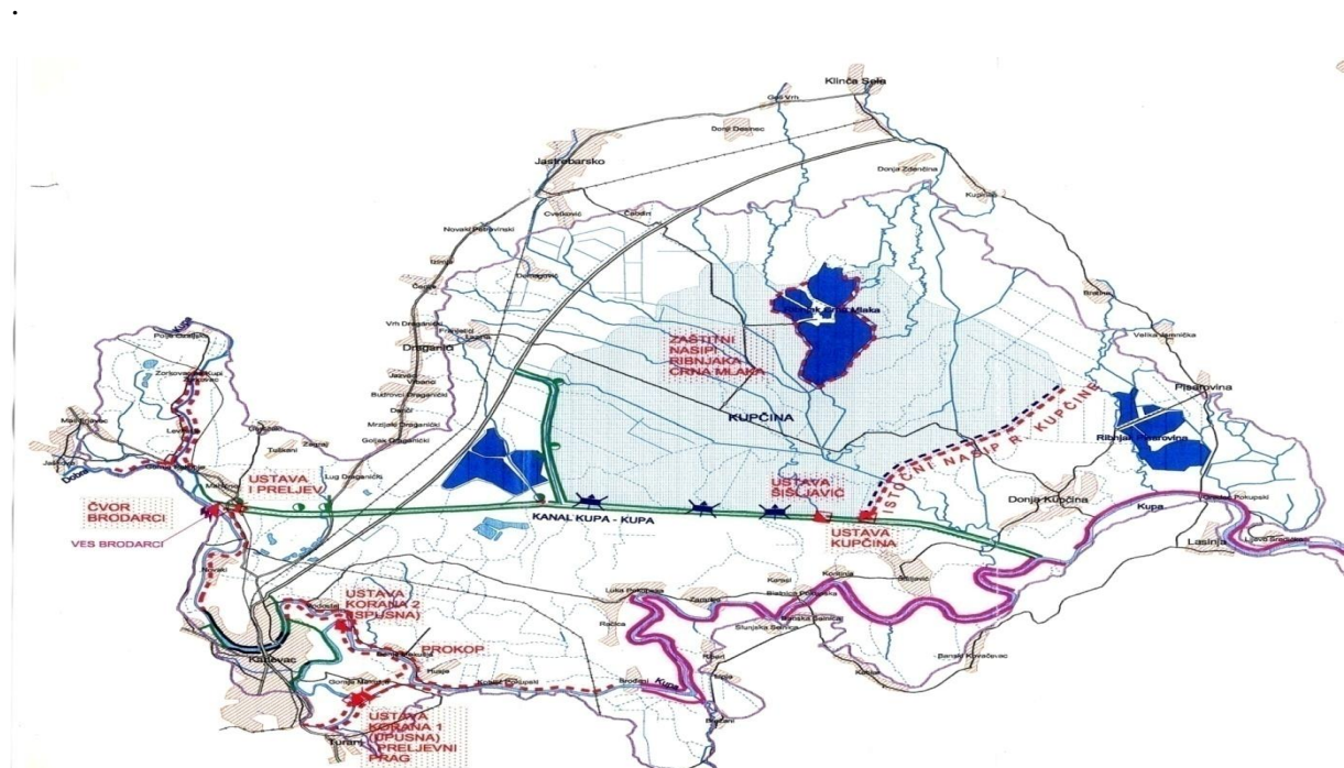
Shema br.2. Konceptija sustava obrane od poplava grada Karlovca
