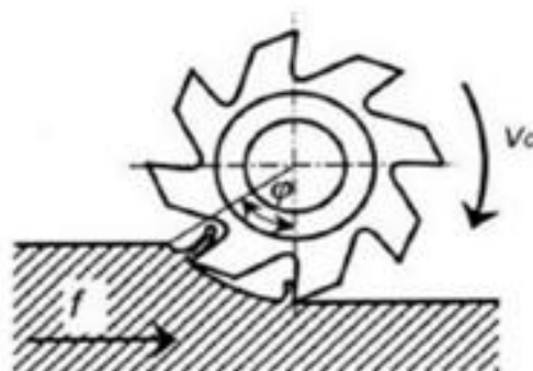
Slika 3. Obodno glodanje
