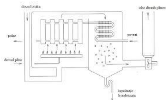
Slika 2: Cijevna grijala
