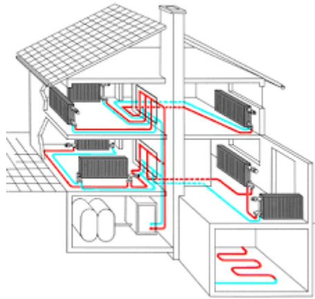
Slika 13: Jednocjevni sustav grijanja
