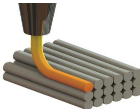
Slika 9. FDM postupak [9]
