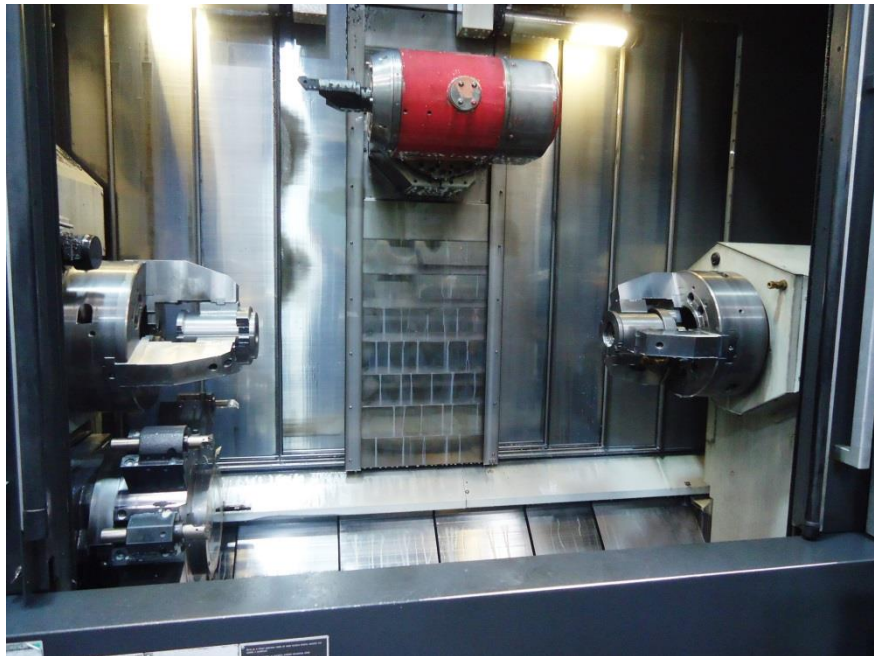
Slika 33. Unutarnje takarenje
