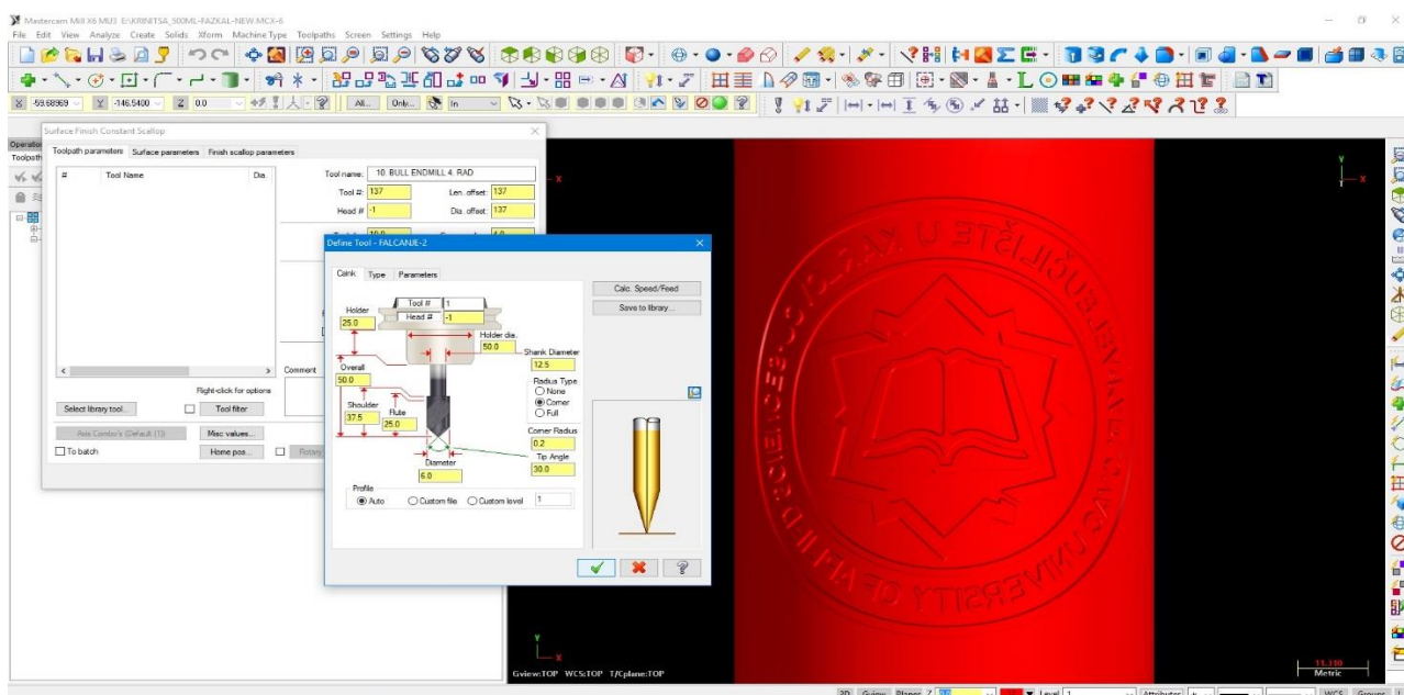
Slika 91. Glodalo za finu obradu definirano unutar Mastercama
