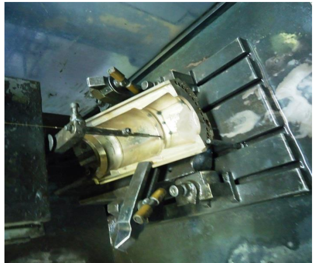
Slika 41. Strojno bušenje vakuum rupica
