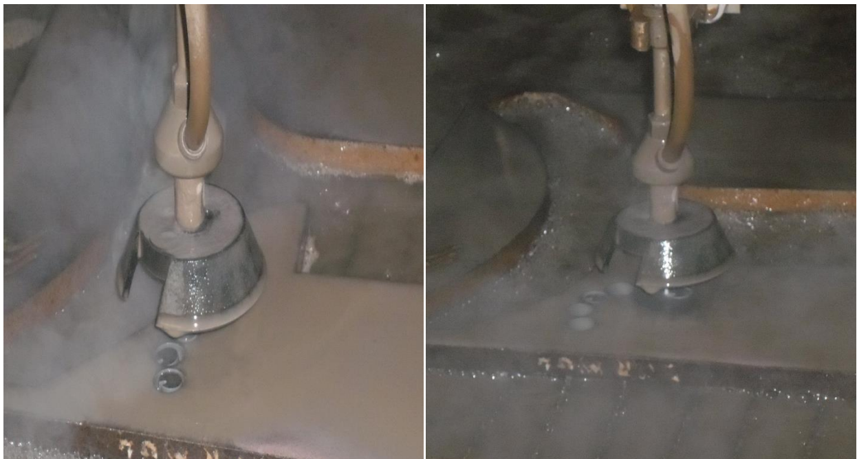
Slika 43. Rezanje provrta promjera 14 mm
