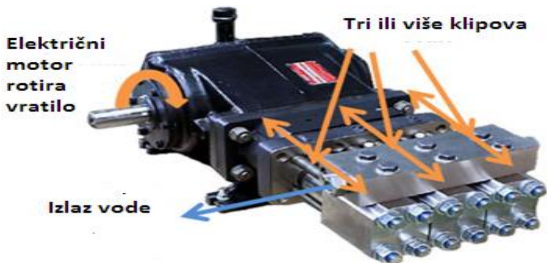
Slika 8. Klipna pumpa
