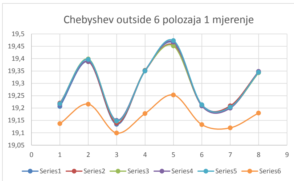
Slika 134. Chebyshev outside za 6 položaja (1 mjerjenje)
