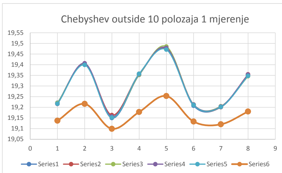
Slika 135. Chebyshev outside za 10 položaja (1 mjerjenje)
