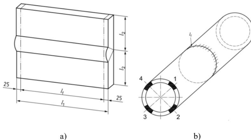
Slika 29. Ispitne dužine za sučeonne zavare: a) za ispitivanje loma na ploči ( l_1 – dužina ispitnog uzorka, l_2 – pola širine ispitnog uzorka, l_f – ispitna dužina); b) za ispitivanje loma i savijanja na cijevi [16]
