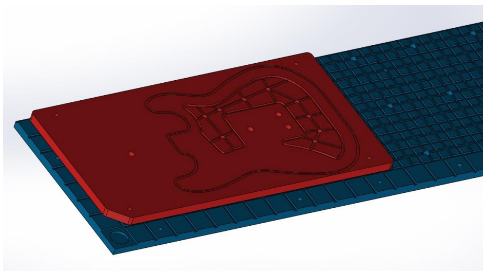
Slika 127. Dopršeni model šablone za tijelo gitare
