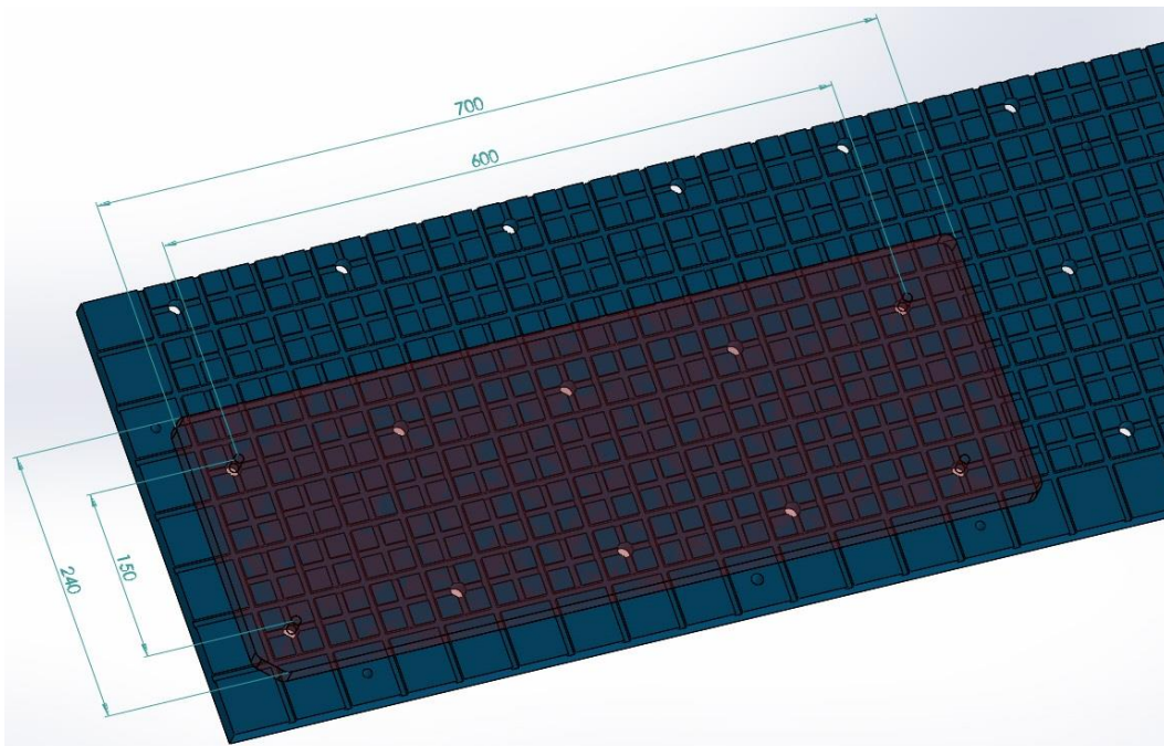
Slika 126. Početak izrade 3D modela šablone za vrat gitare
