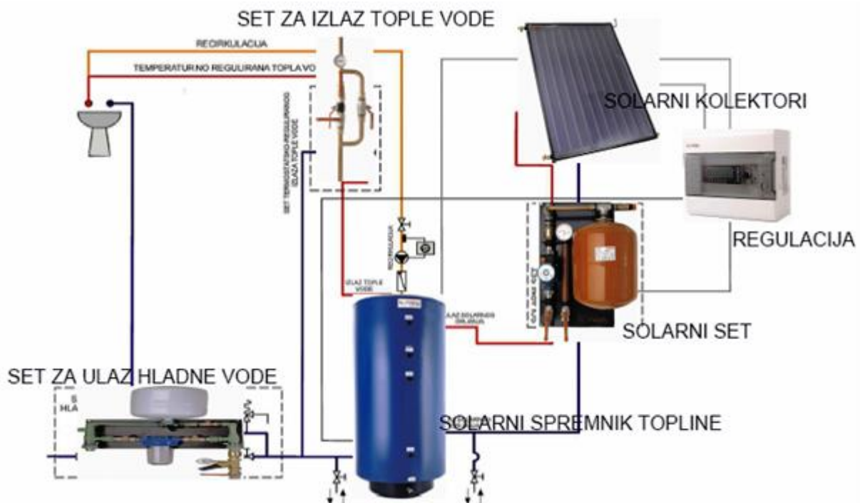
Slika 2. 4. Solarni sustav za pripremu PTV-a
