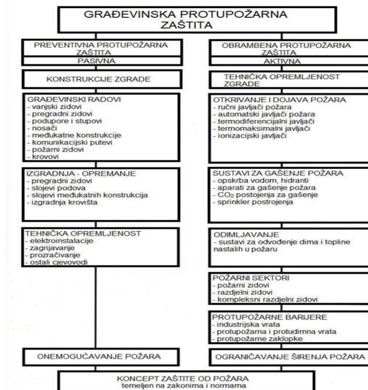
Slika 3. Koncept zaštite od požara [5]
