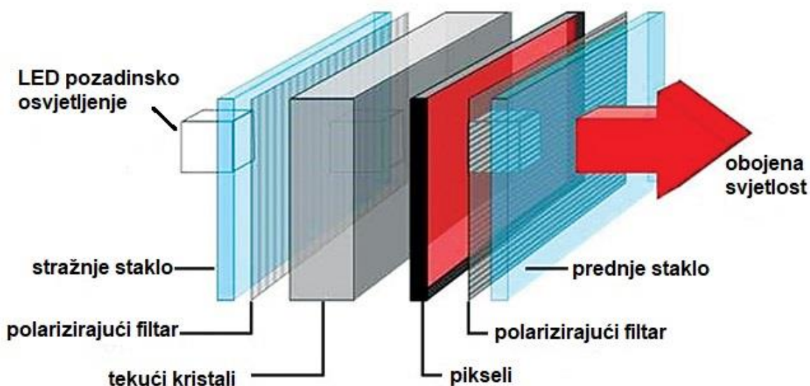
Sl. 5. Građa LED zaslona [11]
