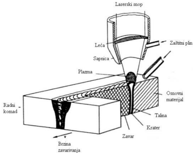
Slika 17. Zavarivanje protaljivanjem
