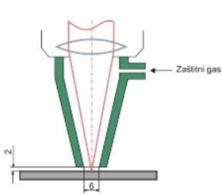
Slika 19. Koaksijalna mlaznica
