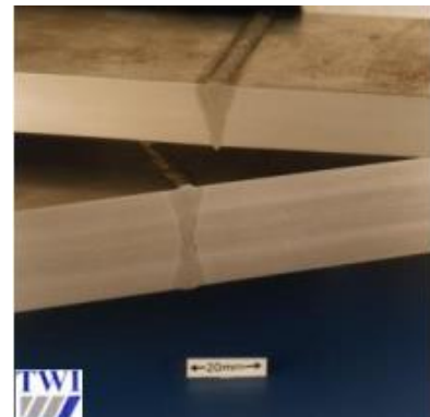
Slika 23. Zavarivanje debljeg lima
