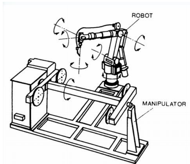
Slika 30. Stupnjevi slobode robota
