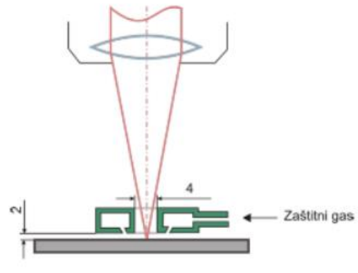
Slika 20. Prstenasti uređaj
