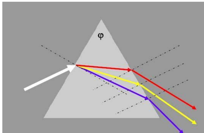
Slika 5. Monokromatska svjetlost
