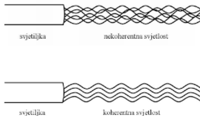
Slika 6. Razlika koherentne i nekoherentne svjetlosti
