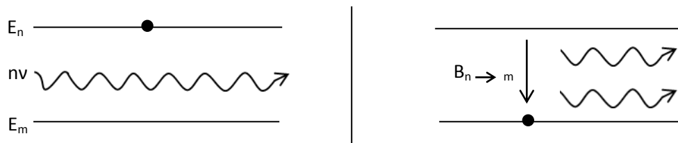
Slika 4. Stimulirana emisija
