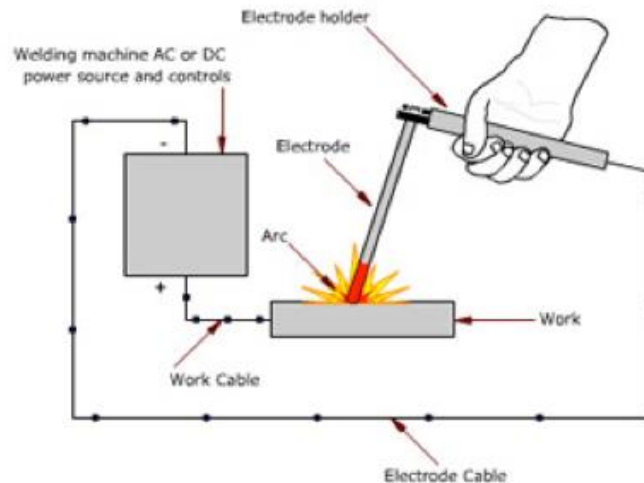
Slika 27. REL postupak zavarivanja
