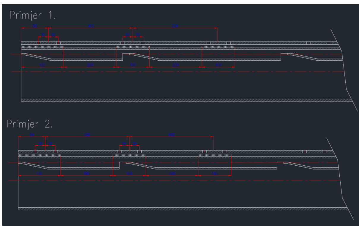
Slika 32. „Novi način” zavora BAR-a na unutarnju cijev
