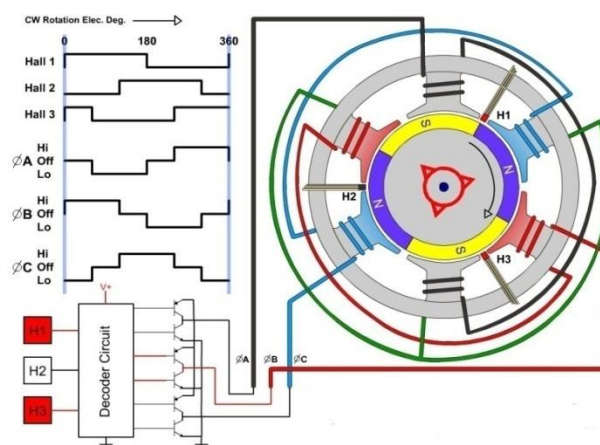
Slika 10: Shema bez kolektorskog motora [10]
