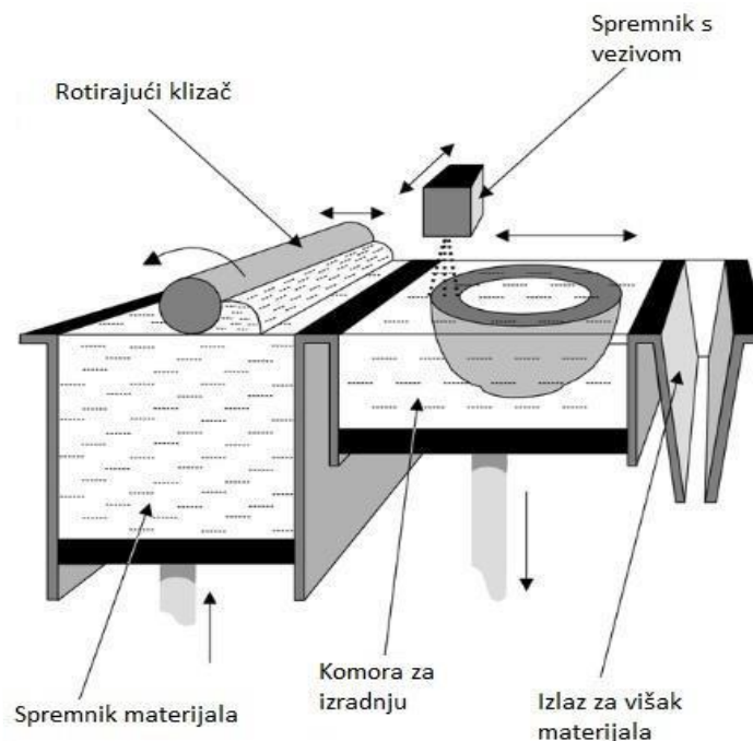
Slika 3.11. Shematski prikaz proizvodnje dijelova 3D tiskanjem [11]
