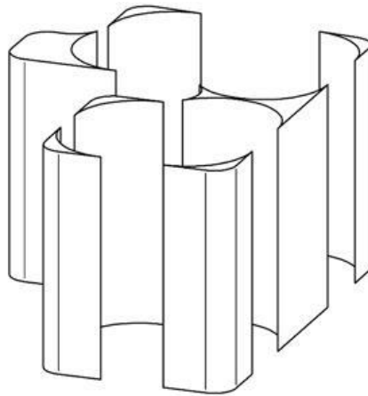
Slika 9: Volumen materijala preostao nakon obrade glodalom Ø35 mm
