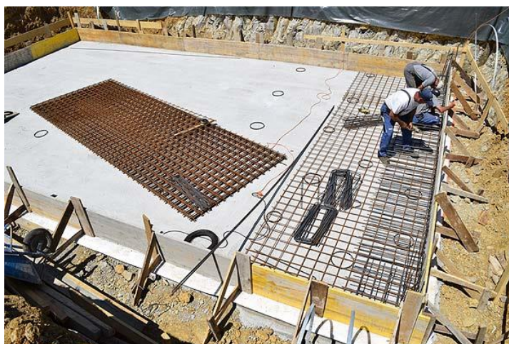
Slika 16. Ugradnja armature [27]
