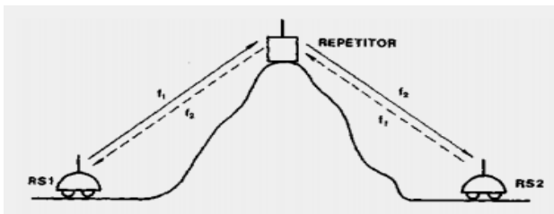
Slika 10. Semidupleksna radiomreža [10]
