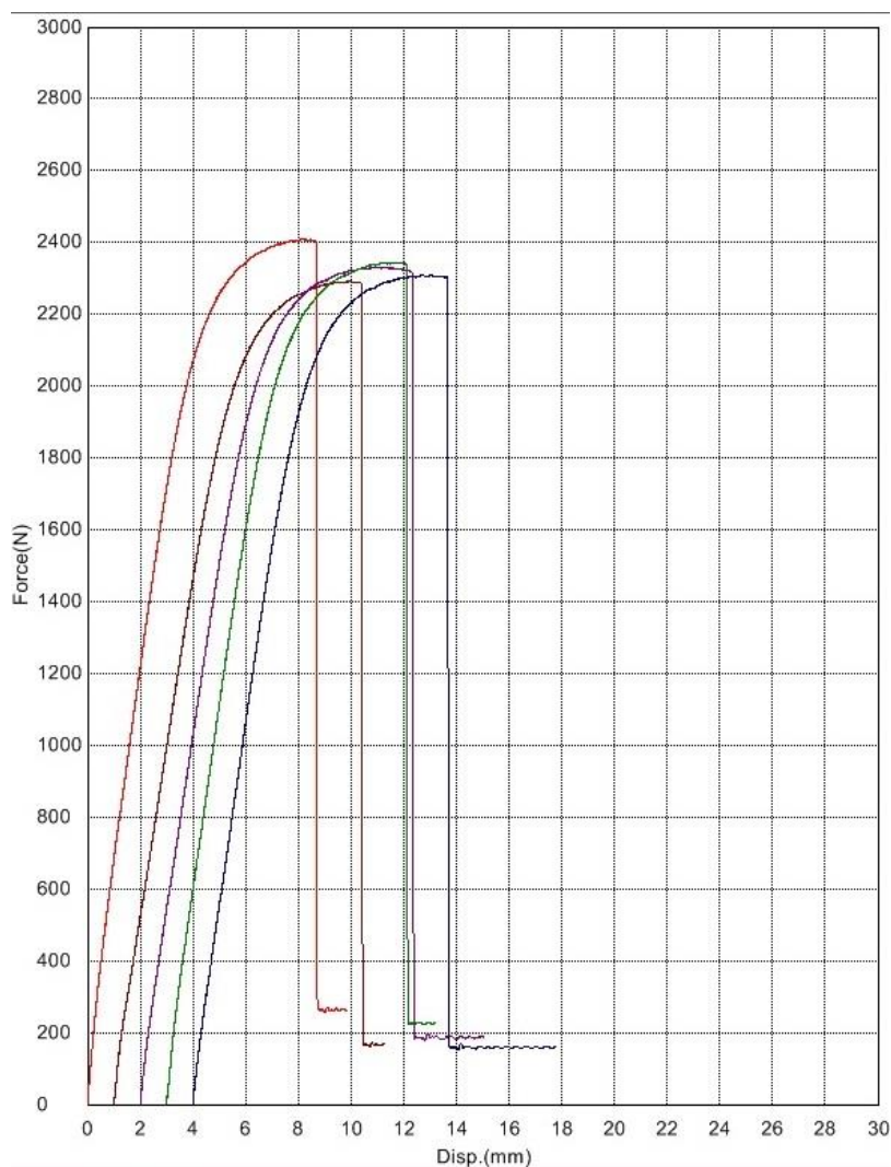
Slika 26. Dijagram napreznosti V epruvete.
