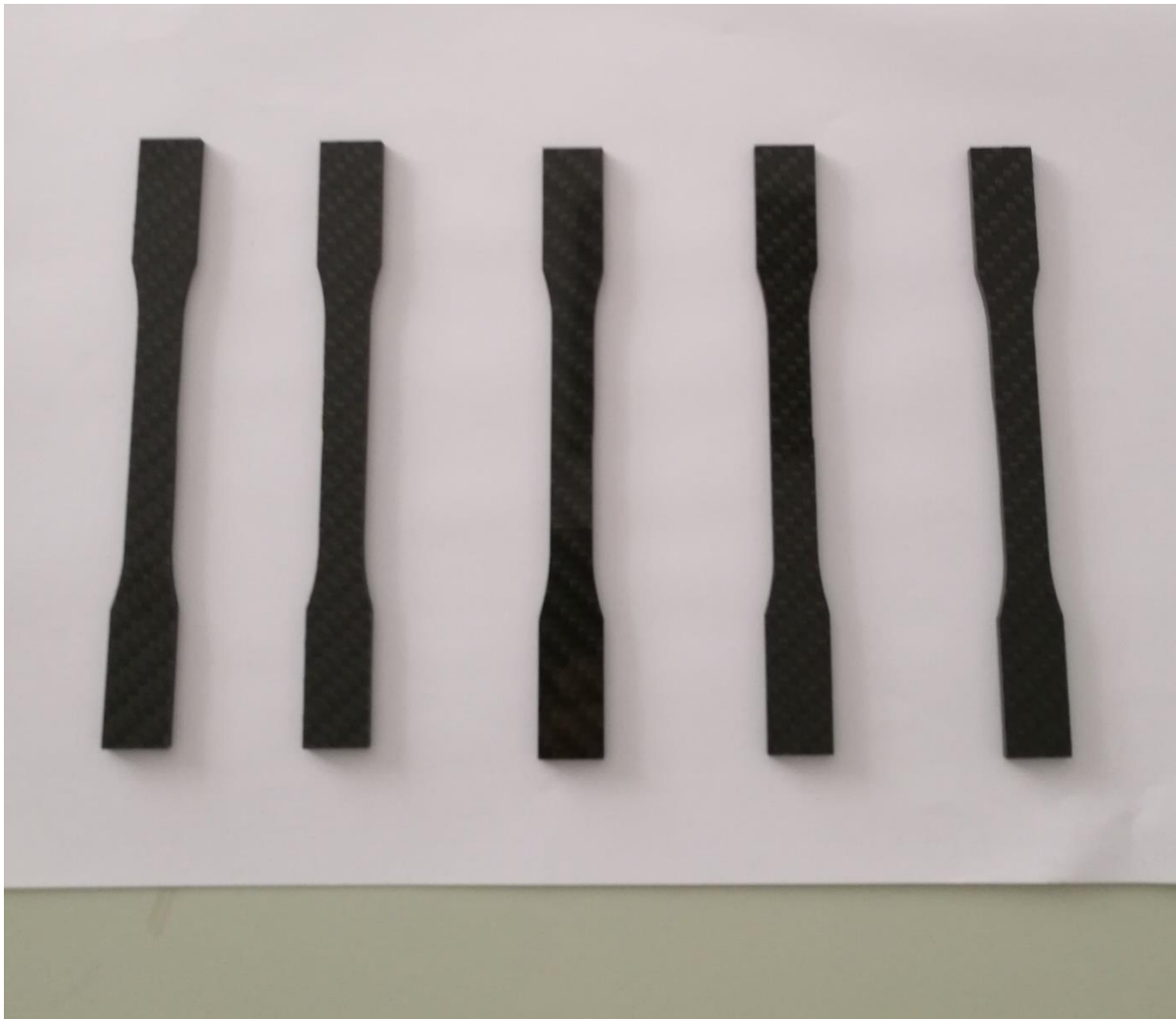
Slika 21. Epruvete pripravljene za ispitivanje vlačne čvrstoće
