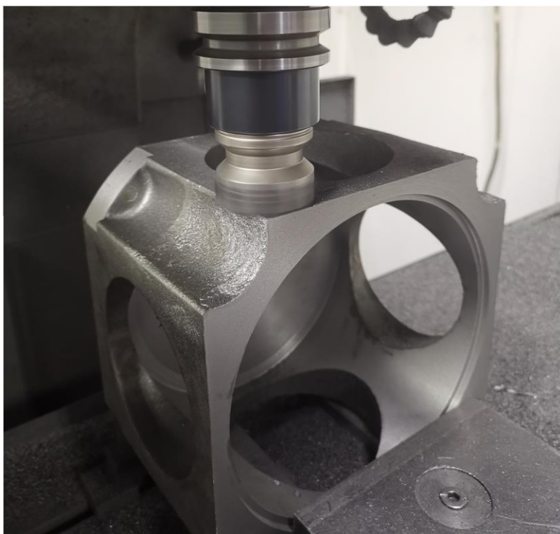
Slika 15. Čeono glodanje
