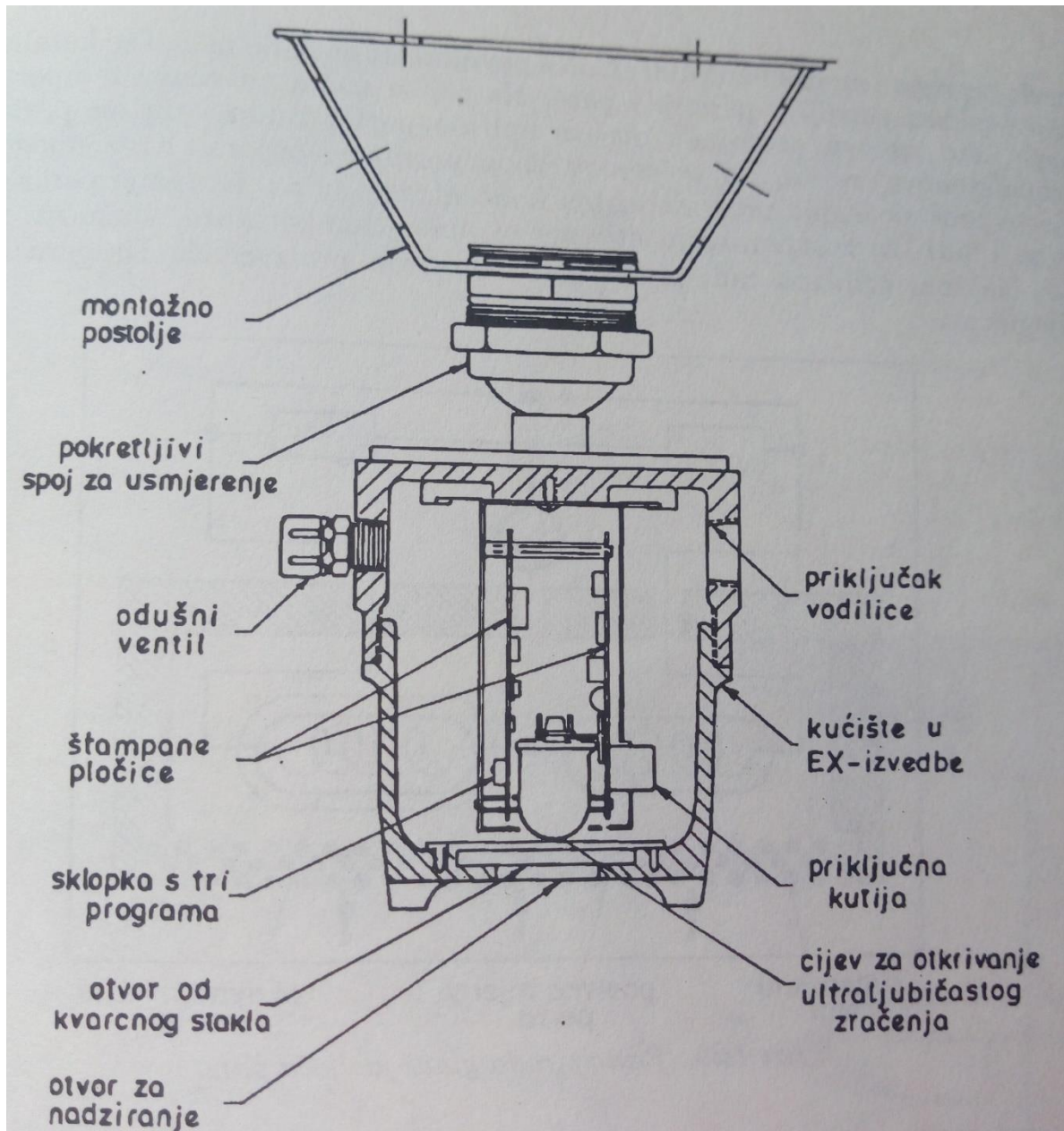
Slika 14. – Predodžba - Ultraljubičasti detektor plamena (5)
