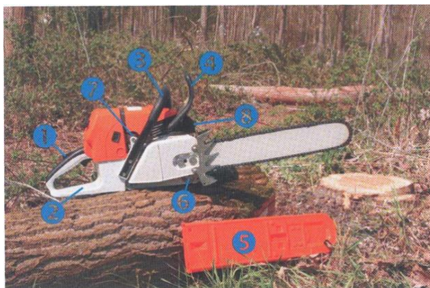
Slika 1 - Zaštitne naprave na motornoj pili
