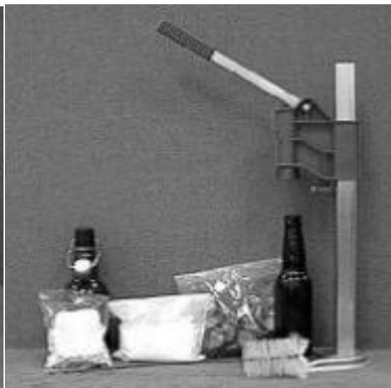
Slika 7. Oprema za flaširanje (Palmer, 2006.)
