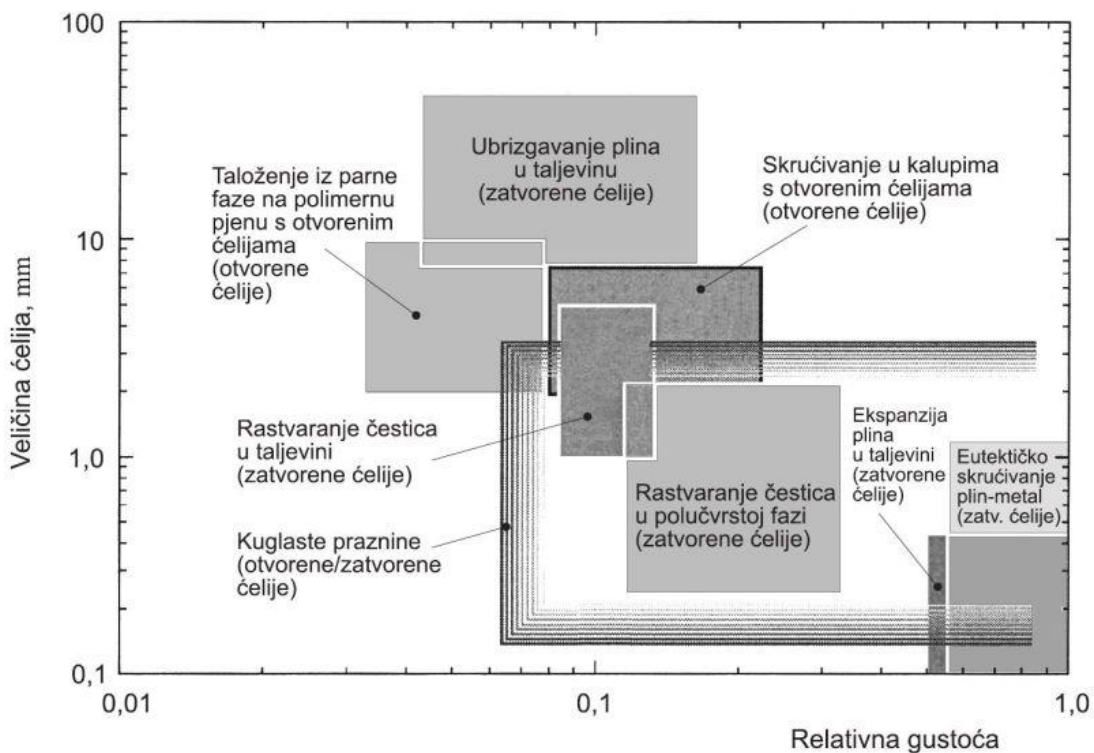
Slika 3. Vrijednosti veličine ćelija i relativne gustoće koje se mogu dobiti određenim proizvodnim postupkom [1]
