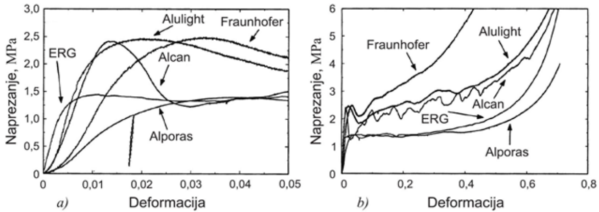
Slika 23. Krivulje “naprezanje-deformacija” pod tlačnim opterećenjem aluminijskih pjena;
