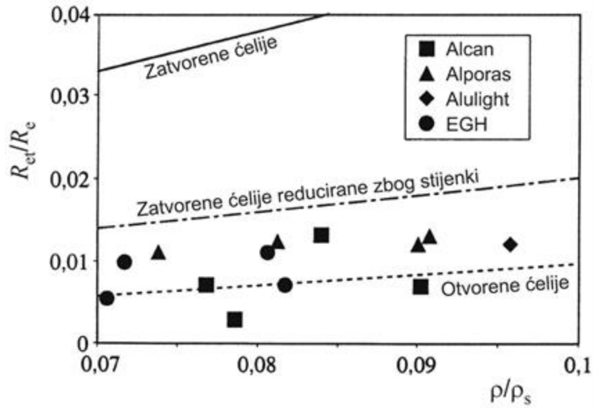
Slika 25. Ovisnost omjera granice stlačivanja pjene ( R_{et} ) i granice tečenja materijala ćelija ( R_c ) [1]
