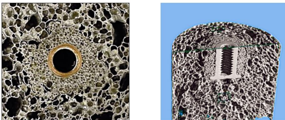
Slika 39. Komadi metalne pjene s bakrenim umetkom [1]
