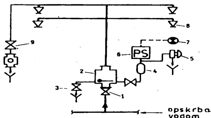
Sl. 2. Mokri sprinkler sustav – dijelovi [13]
