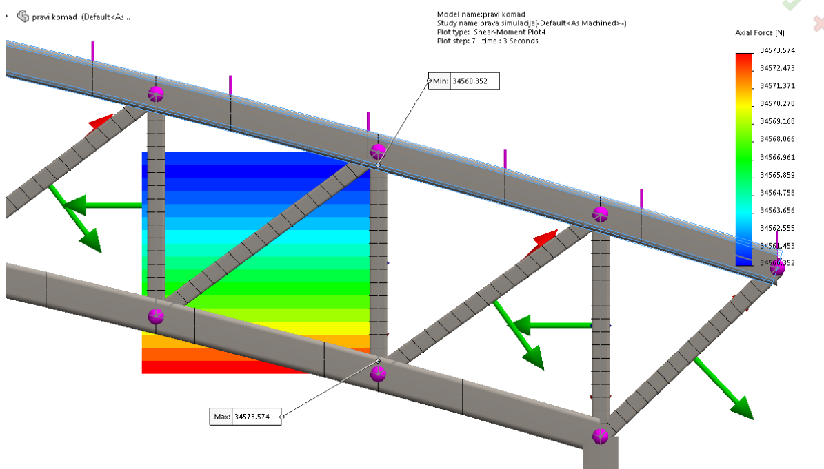
Slika 14 - Aksijalna sila u kritičnom vertikalnom rebrenom štapu
