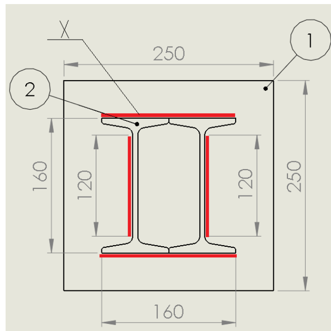
Slika 24 – Geometrijske značajke zavarava ploče i dva stupa
