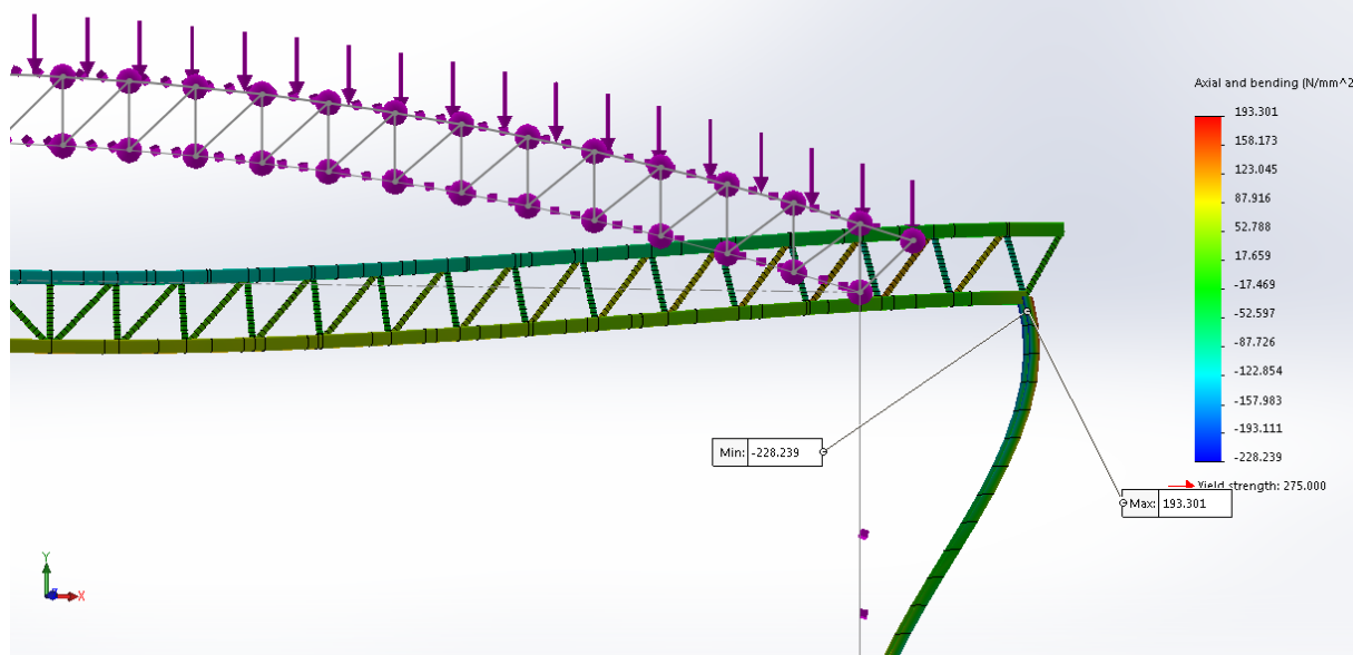
Slika 8 - Ekvivalentna naprezanja s utjecajem vjetrova
