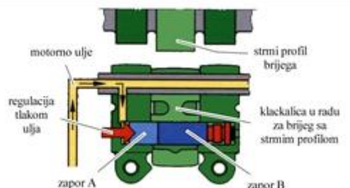
Slika 9. Pokretanje ventila na visokom broju okretaja
