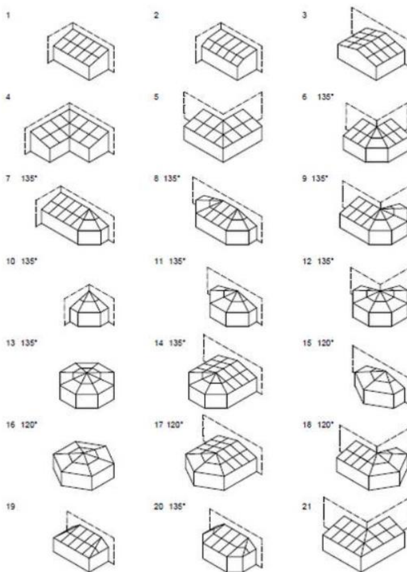
Slika 15. Moguće varijante izvedbe zimskih vrtova
