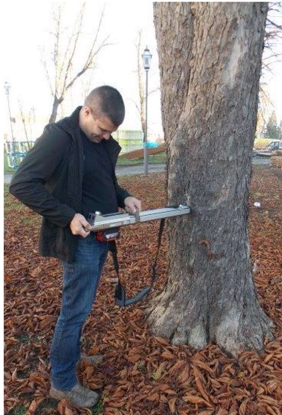
Slika br. 8 Rezistograf daje uvid u stanje debla stabla
