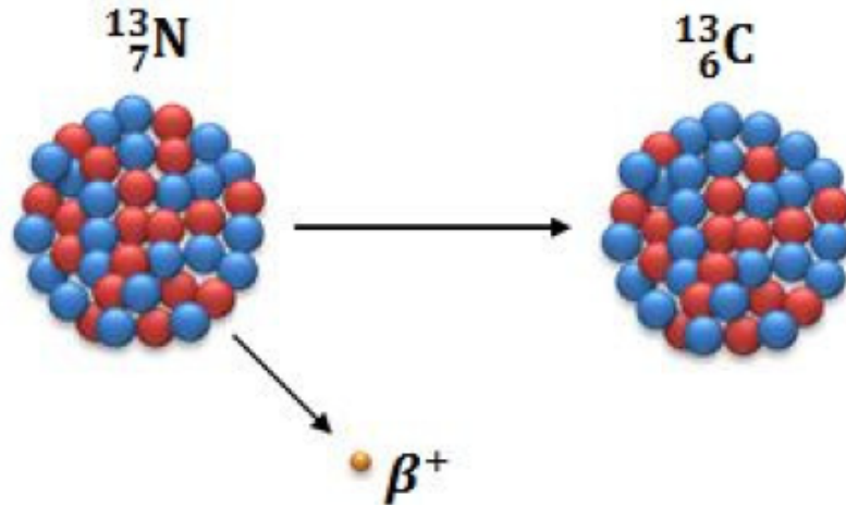
Slika 9: Raspad N-13
