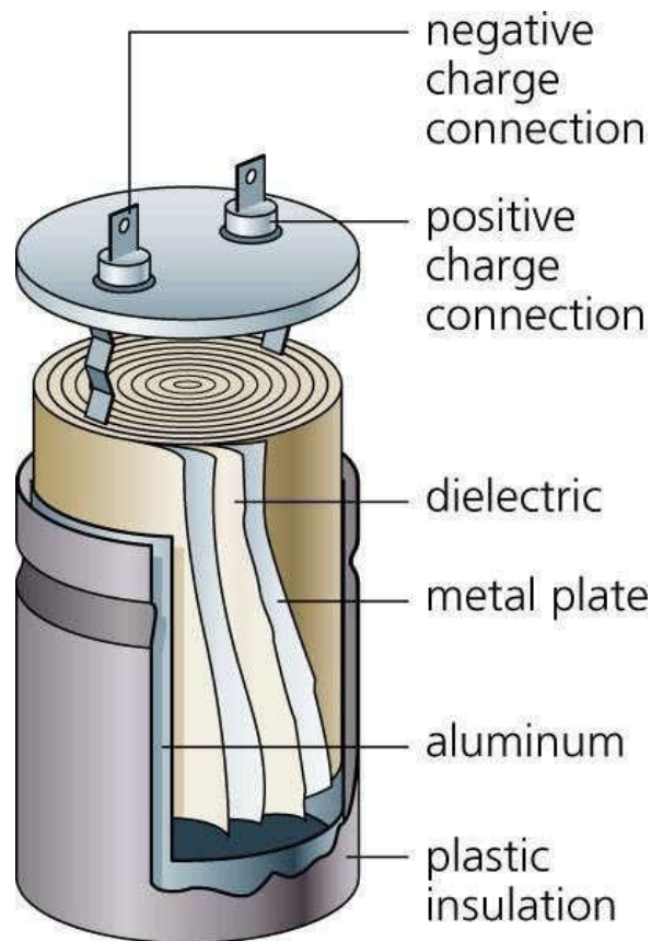
Slika 14. Unutrašnjost kondenzatora
