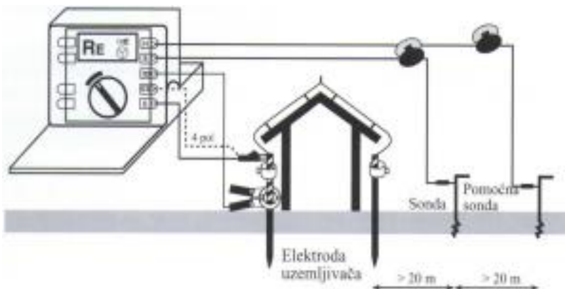
Slika 27. Predodžba mjerenje otpora uzemljenja pomoću strujnih kliješta i sondi [14]
