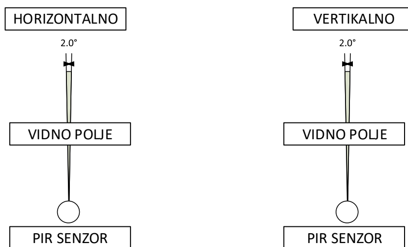
Slika 11. Prikaz vidnog polja senzora bez fresnelove leće i kada je snop ograničen termalno otpornom barijerom (sigurnosna zraka za detekciju pokreta)
