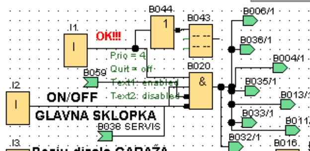
Slika 40. I1 OK!!! i I2 ON/OFF GLAVNA SKLOPKA
