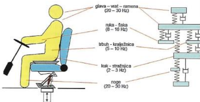
Slika 24. Prijenos vibracija
