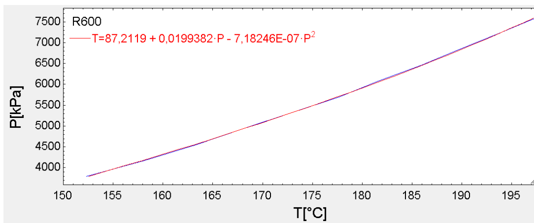
Slika 4-62: Prikaz ovisnosti pseudokritične temperature o nadkritičnom tlaku za radni fluid R600
