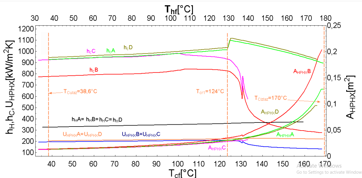
Slika 4-100: Prikaz promjene vrijednosti koeficijenta prijelaza toplote ( h_H, h_C ), ukupnih koeficijenta prolaza toplote ( U_{HPHX} ) i površina segmenata izmjenjivača toplote ( A_{HPHX} ) duž razmatranog izmjenjivača toplote za radni fluid R236fa
